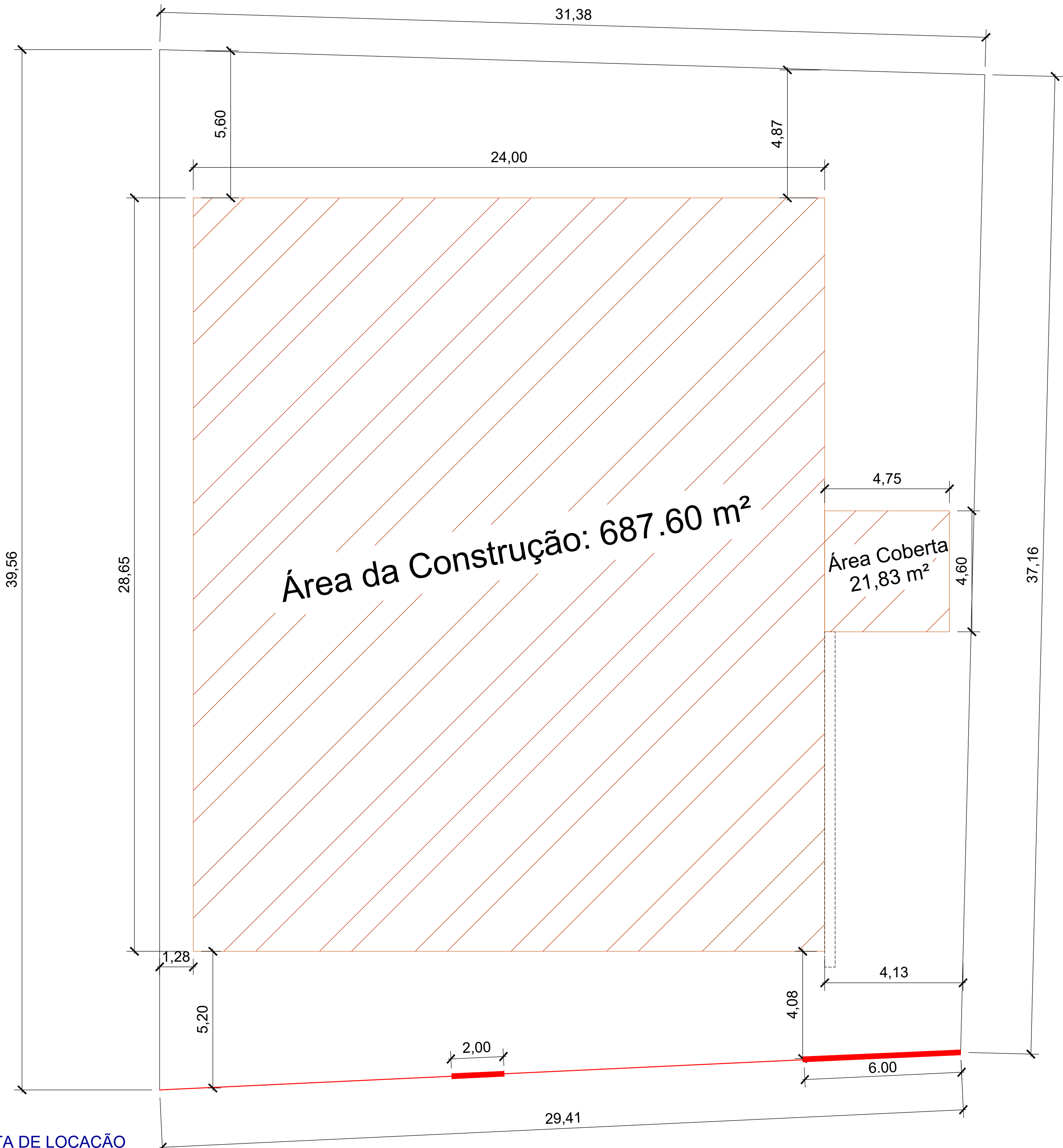
PLANTA DE LOCAÇÃO ESC.: 1/100
